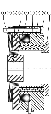
BRAKE SERIE K/BFK
