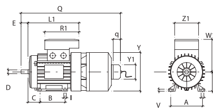
BAE B5
