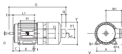
Estremità d'albero
